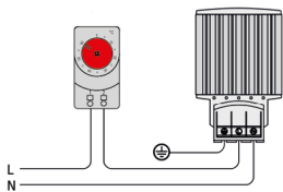
Thermostat KTO 111 (NC)
