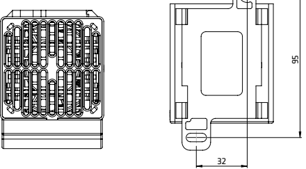
Fan Heater CS 028
